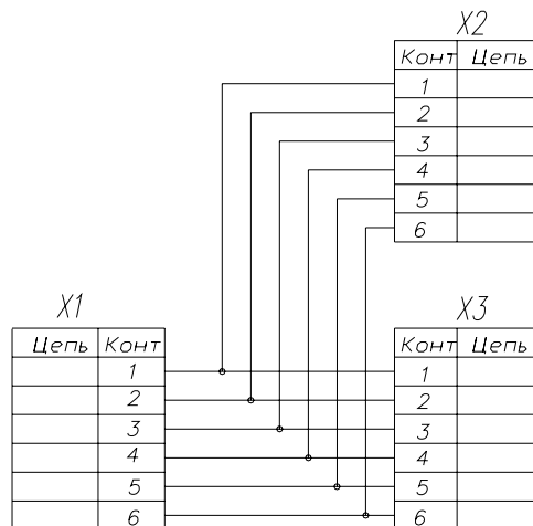
Рис. 1. РП-3-У. Схема электрическая принципиальная.
